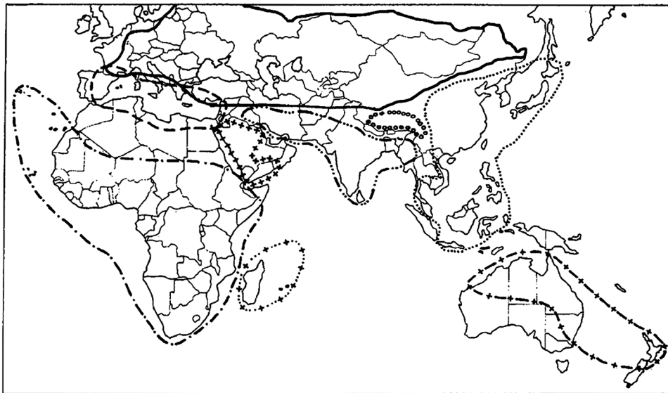
Fig. 7 Distribution range of the races/subspecies of the migratory locust Locusta migratoria L. (modified from Refs. 30, 32, and 33). Locusta m. migratoria and L. m. rossica —; L. m. cinerascens - - -; L. m. burmana •••••; Indian subspecies •••—; L. m. migratorioides —•—•—; L. m. capito +•••+; Arabian subspecies +++; L. m. manilensis ....; Australian subspecies -++-.
